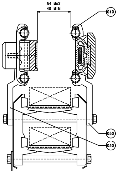
D - D, B55
