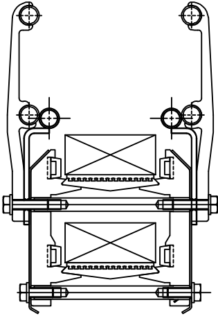
A - A, 1:1
