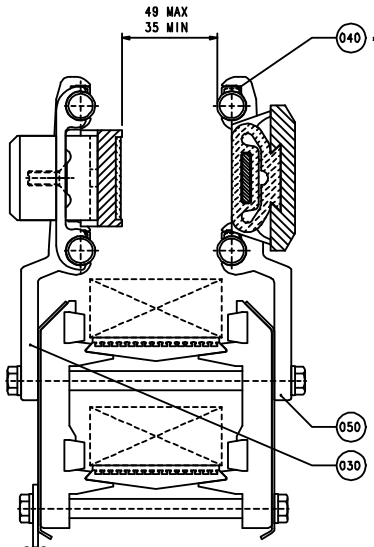
D - D, B50
