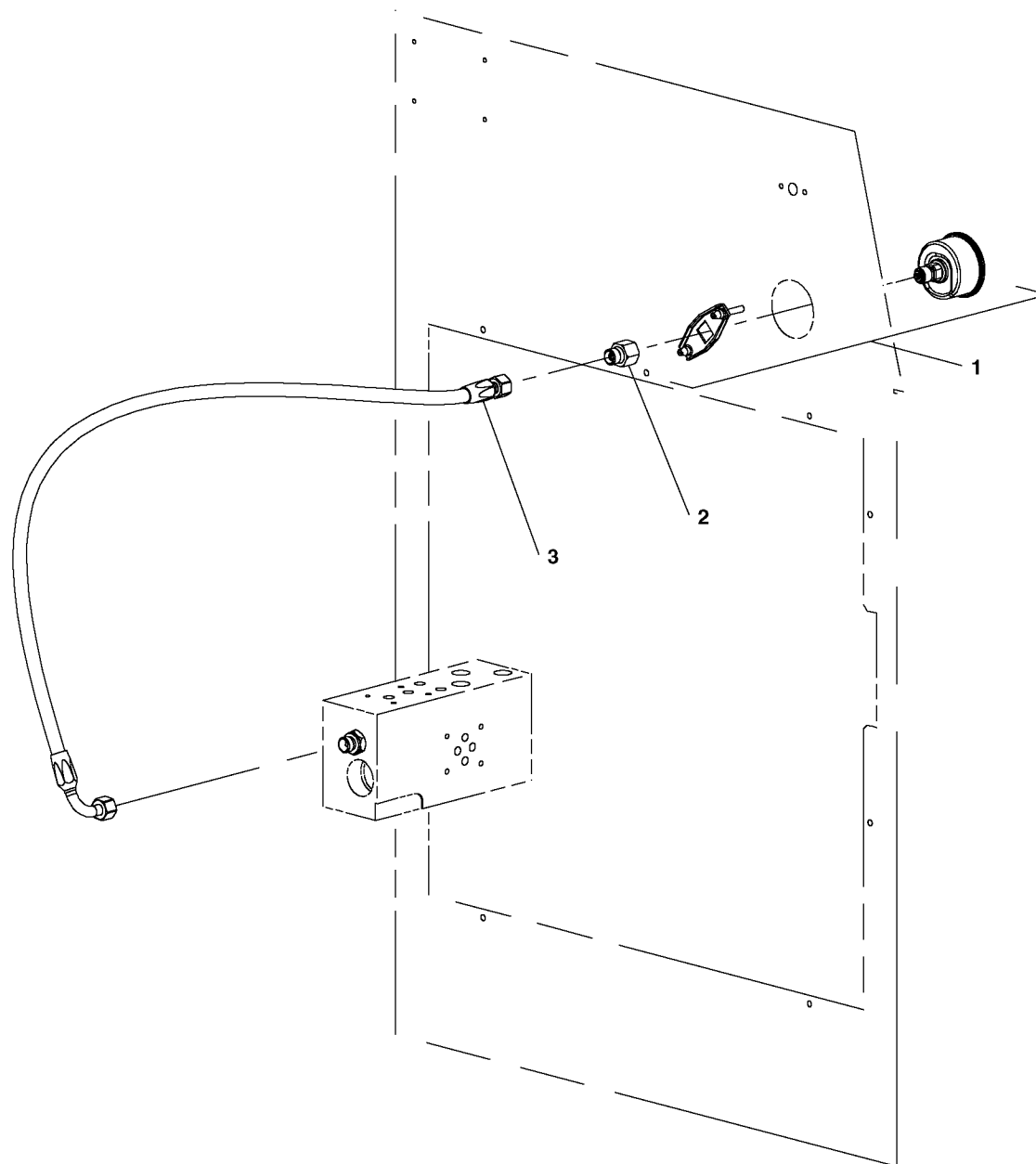
MANOMETER
